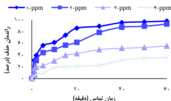
شکل ۶. تأثیر غلظت رنگ (RB-5) در کارایی نانوذرات جهت حذف رنگ
