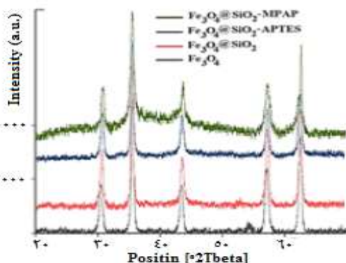
شکل ۳. نمای XRD (X-Ray Diffraction) از نانوذرات مغناطیسی
