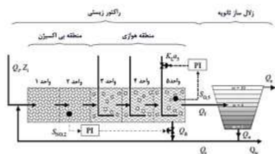
شکل ۱. نمای شماتیک Benchmark Simulation Model No. 1 (BSM1) (۸)
