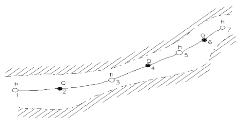
شکل ۱. شماتیک گره‌بندی رودخانه در مدل MIKE ۱۱ (۷)
