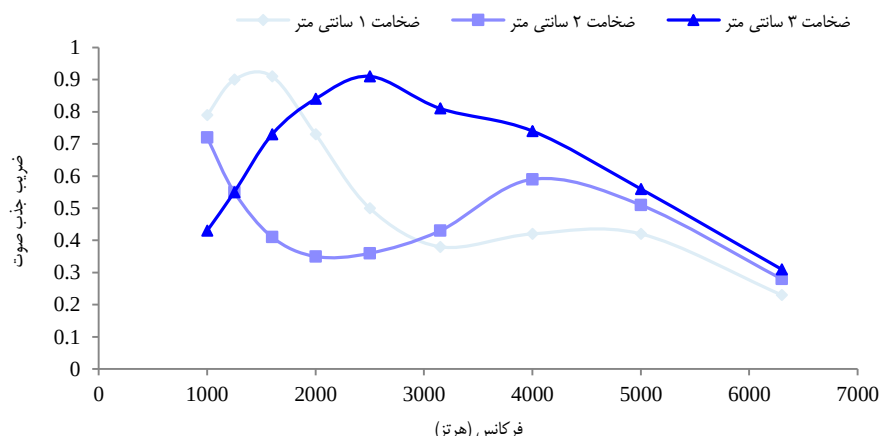
شکل ۶. طیف جذب پیل‌های خمیر کاغذ با چگالی ۳۵۰ کیلوگرم بر مترمکعب در ضخامت‌های مختلف
