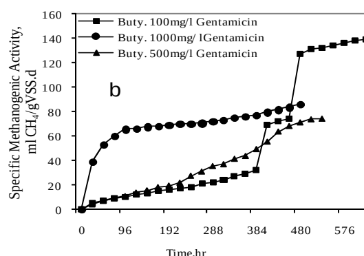
نمودار ۴: تأثیر آننتی بیوتیک‌های آمپی‌سیلین و جنتامایسین بر روی میزان تجمعی متان‌سازی ویژه بیومس بی‌هوازی (الف): غلظت‌های متفاوت آمپی‌سیلین بر روی بوتیریک اسید شامل ۱۰۰۰ (●)، ۵۰۰ (▲) و ۲۰۰ (■) میلی‌گرم در لیتر و (ب) غلظت‌های متفاوت جنتامایسین بر روی بوتیریک اسید شامل ۱۰۰۰ (●)، ۵۰۰ (▲) و ۱۰۰ (■) میلی‌گرم در لیتر (کلمه اختصار Buty. در نمودارها به معنی بوتیریک اسید است)
