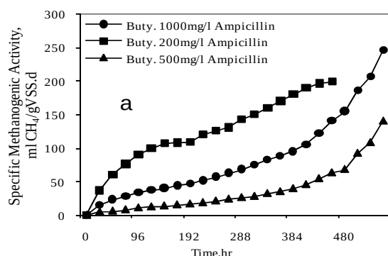
نمودار ۴: تأثیر آننتی بیوتیک‌های آمپی‌سیلین و جنتامایسین بر روی میزان تجمعی متان‌سازی ویژه بیومس بی‌هوازی (الف): غلظت‌های متفاوت آمپی‌سیلین بر روی بوتیریک اسید شامل ۱۰۰۰ (●)، ۵۰۰ (▲) و ۲۰۰ (■) میلی‌گرم در لیتر و (ب) غلظت‌های متفاوت جنتامایسین بر روی بوتیریک اسید شامل ۱۰۰۰ (●)، ۵۰۰ (▲) و ۱۰۰ (■) میلی‌گرم در لیتر (کلمه اختصار Buty. در نمودارها به معنی بوتیریک اسید است)
