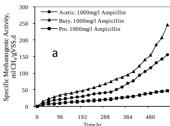
نمودار ۷: تأثیر آنتی بیوتیک‌های آمپی سیلین و جنتامایسین بر روی میزان تجمع متان‌سازی ویژه بیومس بی‌هوازی: (الف): غلظت ۱۰۰۰ میلی گرم در لیتر آمپی سیلین بر روی سه نوع اسید چرب شامل استیک اسید (●)، بوتیریک اسید (▲) و پروپیونیک اسید (■) و (ب) غلظت ۱۰۰۰ میلی گرم در لیتر جنتامایسین بر روی سه نوع اسید چرب شامل استیک اسید (●)، بوتیریک اسید (▲) و پروپیونیک اسید (■)
