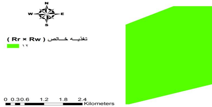
شکل ۲. لایه تغذیه خالص آبخوان موجود در مکان دفن پسماند اصفهان
