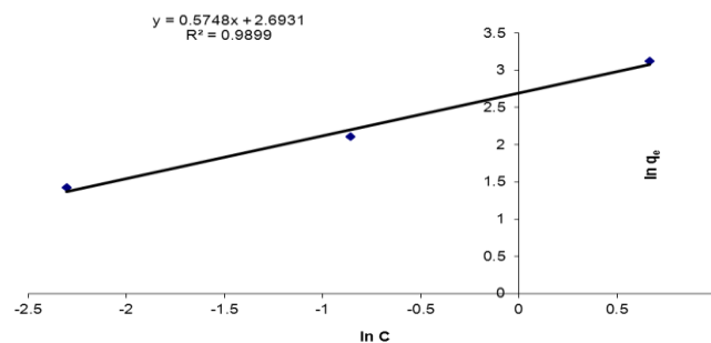
نمودار ۹. ایزوترم فروندلیچ نانولوله کربنی تک‌جداره با دوز جاذب ۰/۱، ۰/۳، ۰/۶، ۰/۹ گرم در لیتر (زمان ۲۴ ساعت و در pH=۴ و غلظت اولیه رنگ ۲۵ میلی‌گرم در لیتر)
