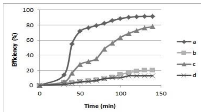
شکل ۷. راندمان حذف کاتالیستی با 3/9\text{ w/m}^2 شدت تابش فرابنفش (a) TiO_2/Z\text{eolite} با غلظت 10\text{ mg/L} (b) TiO_2 با غلظت 10\text{ mg/L} : (c) TiO_2/Z\text{eolite} با غلظت 50\text{ mg/L} (d) TiO_2 با غلظت 50\text{ mg/L}
