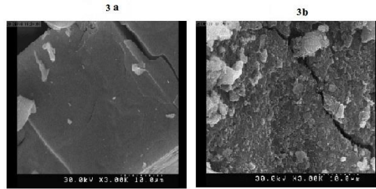
شکل (a) ۳. الگوی SEM نانوذرات TiO_2 - شکل (b) ۳- الگوی SEM TiO_2/Zeolite
