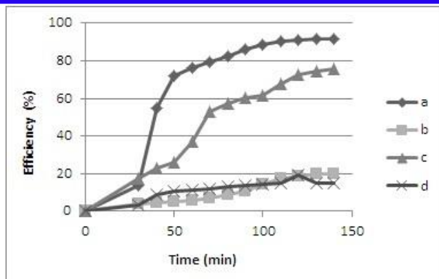
شکل ۵. راندمان حذف فتوکاتالیستی با غلظت 10\text{ mg/L} (a) TiO_2/Z\text{eolite} با شدت تابش 3/9\text{ w/m}^2 (b) TiO_2 با شدت تابش 3/9\text{ w/m}^2 : (c) TiO_2/Z\text{eolite} با شدت تابش 2/4\text{ w/m}^2 (d) TiO_2 با شدت تابش 2/4\text{ w/m}^2
