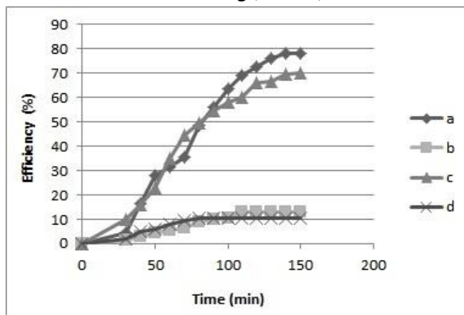
شکل ۶. راندمان حذف فتوکاتالیستی با غلظت 50\text{ mg/L} (a) TiO_2/Z\text{eolite} با شدت تابش 3/9\text{ w/m}^2 (b) TiO_2 با شدت تابش 3/9\text{ w/m}^2 : (c) TiO_2/Z\text{eolite} با شدت تابش 2/4\text{ w/m}^2 (d) TiO_2 با شدت تابش 2/4\text{ w/m}^2
