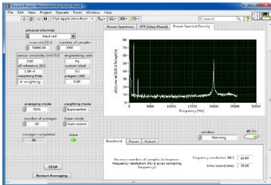
شکل ۱۱. نتایج اندازه گیری تراکم طیف توان صوت
