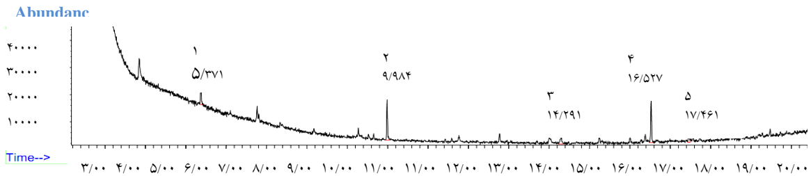
شکل ۱. کروماتوگرام مواد حد واسط تشکیل شده بعد از ۱۰ دقیقه ازن زنی تحت شرایط بهینه
