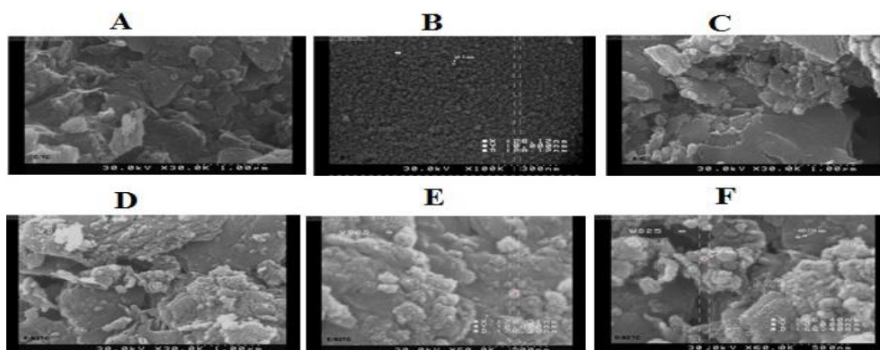
شکل ۲. تصاویر SEM نمونه‌های A: C (Clinoptilolite)؛ B: T_1 ( TiO_2 )؛ C: TC ( TiO_2/Cl ) و D، E، F: N_7TC SEM: Scanning electronic microscope
