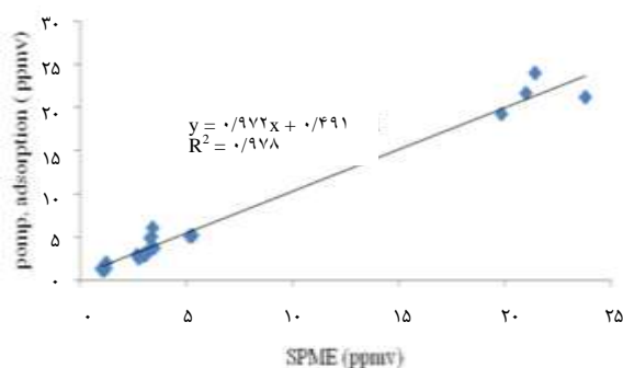
شکل ۱. مقایسه دو روش Solid-phase microextraction (SPME) و پمپ و جذب برای تعیین مقدار بنزن بر اساس نرخ نمونه‌برداری واقعی محاسبه شده
