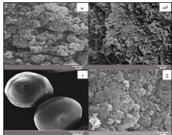
شکل ۲. تصاویر SEM Scanning electron microscopy (الف) کیتوسان خام (الف)، (ب) Carbon Nanotube (CNT) اکسید شده (ب)، (ج و د) Chitosan/Carbon Nanotube (CHN-CNT)
