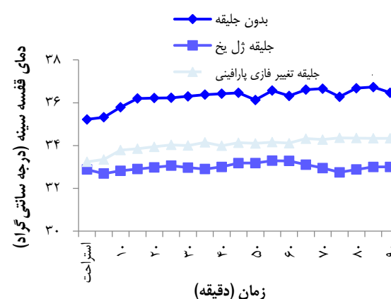
شکل ۵. روند زمانی تغییرات میانگین دمای پوست در ناحیه سینه افراد در سه حالت بدون جلیقه خنک‌کننده، با جلیقه خنک‌کننده ژل یخ و با جلیقه خنک‌کننده تغییر فازی پارافینی
