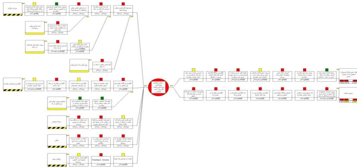
نمودار ۲: نمودار پایبونی پیامد سیلندره‌های تحت فشار، جوشکاری و برشکاری با گاز راهنمای نمودار
