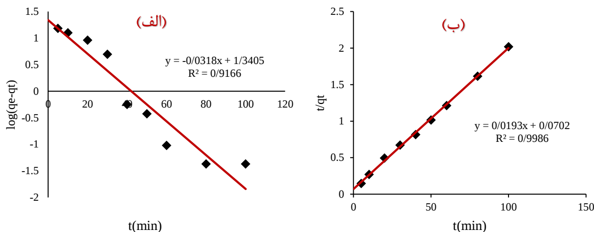
شکل ۷: جذب آنتراسن توسط دندریمر مغناطیسی براساس مدل سینتیکی: (الف) شبه درجه اول؛ (ب) شبه درجه دوم
