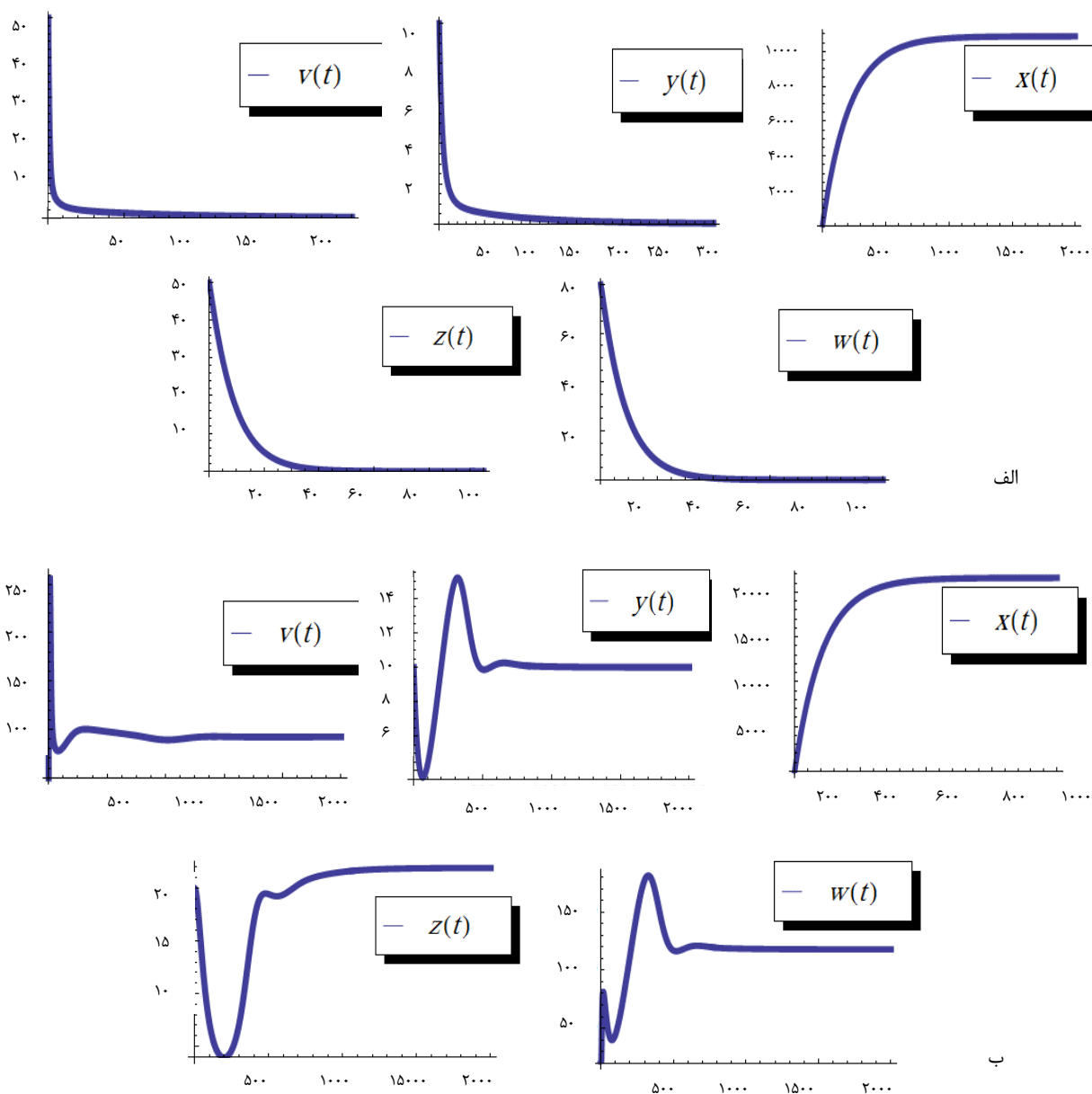
شکل ۵. مدل ریاضی ویروس Human immunodeficiency virus (HIV) در دو حالت R_0 < 1 (الف) و R_0 > 1 (ب)
