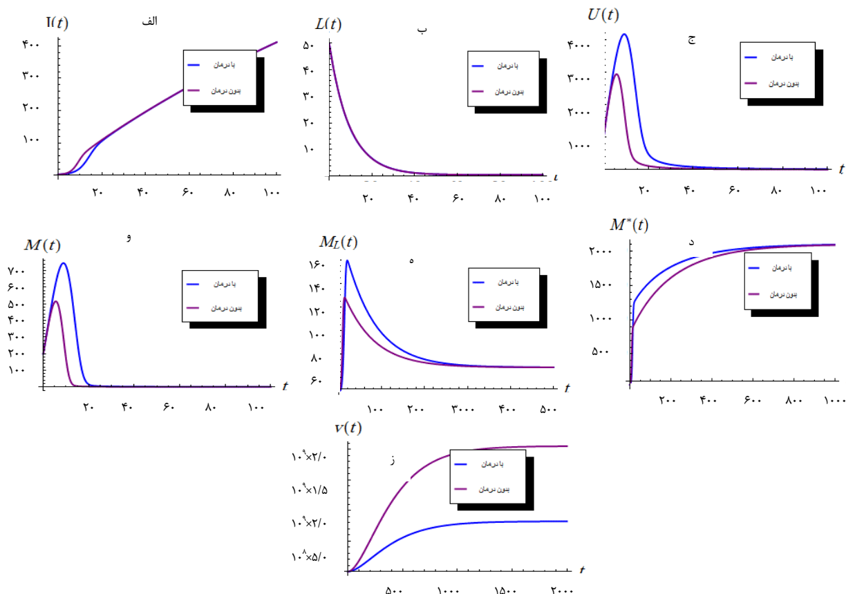
شکل ۶. مقایسه مدل ویروس Human immunodeficiency virus (HIV) در حضور و عدم حضور درمان
