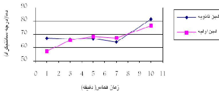
نمودار ۱۲: روند تغییرات دمای نمونه‌های لجن به وزن ۲۰ گرم حاوی ۵ درصد زغال در زمان تماس‌های مختلف در مایکروویو
