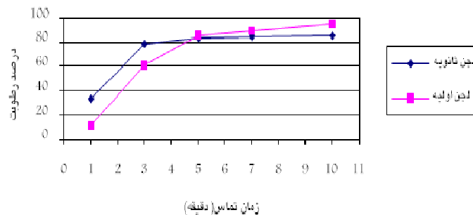
نمودار ۱۴: روند افزایش درصد حذف رطوبت نمونه‌های لجن به وزن ۲۰ گرم حاوی ۵ درصد زغال در زمان تماس‌های مختلف در مایکروویو
