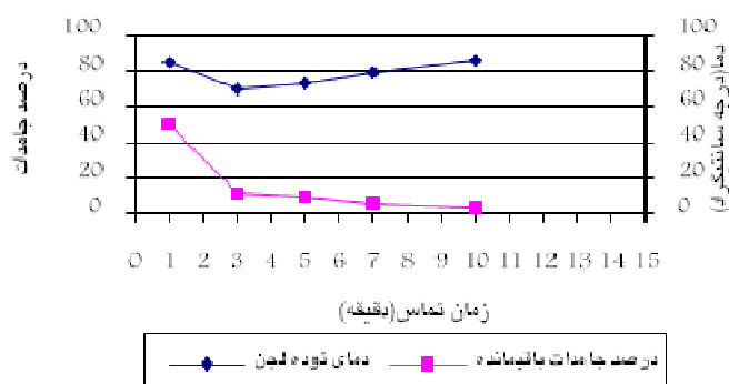
نمودار ۲: کاهش درصد جامدات و افزایش دما در نمونه‌های لجن اولیه به وزن ۲۰ گرم در زمان‌های تماس مختلف در مایکروویو
