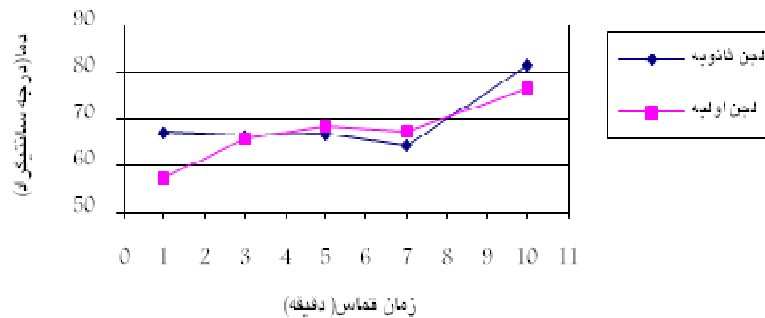
نمودار ۱۲: روند تغییرات دمای نمونه‌های لجن به وزن ۲۰ گرم حاوی ۵ درصد زغال در زمان تماس‌های مختلف در مایکروویو
