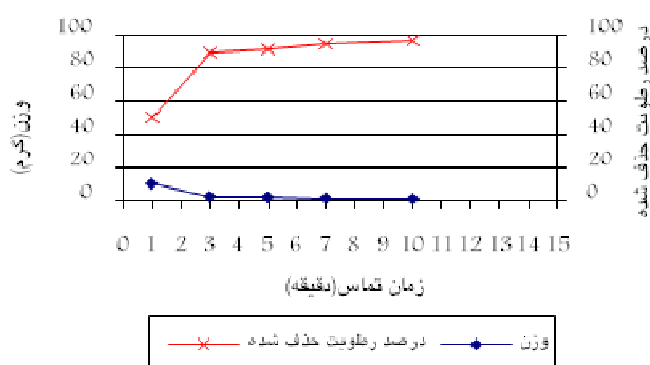
نمودار ۱: کاهش وزن و درصد حذف رطوبت در نمونه‌های لجن اولیه به وزن ۲۰ گرم در زمان‌های تماس مختلف در مایکروویو
