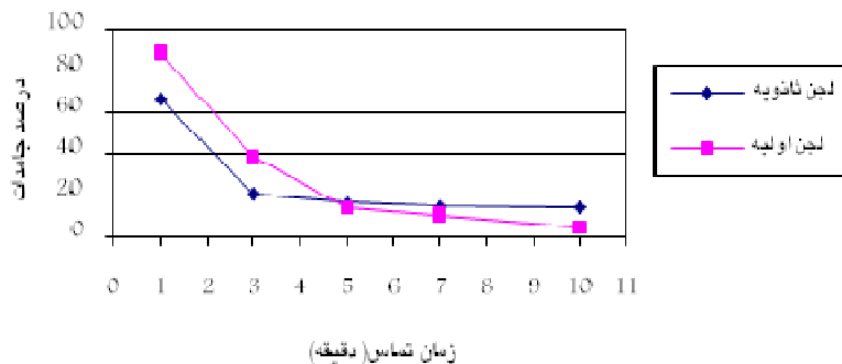
نمودار ۱۳: روند کاهش درصد جامدات نمونه‌های لجن به وزن ۲۰ گرم حاوی ۵ درصد زغال در زمان تماس‌های مختلف در مایکروویو
