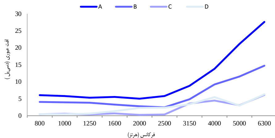
شکل ۱. تغییرات افت عبوری در فرکانس یک سوم اکتاوباند در جاذب چهار گروه گوشی حفاظتی A, B, C و D
