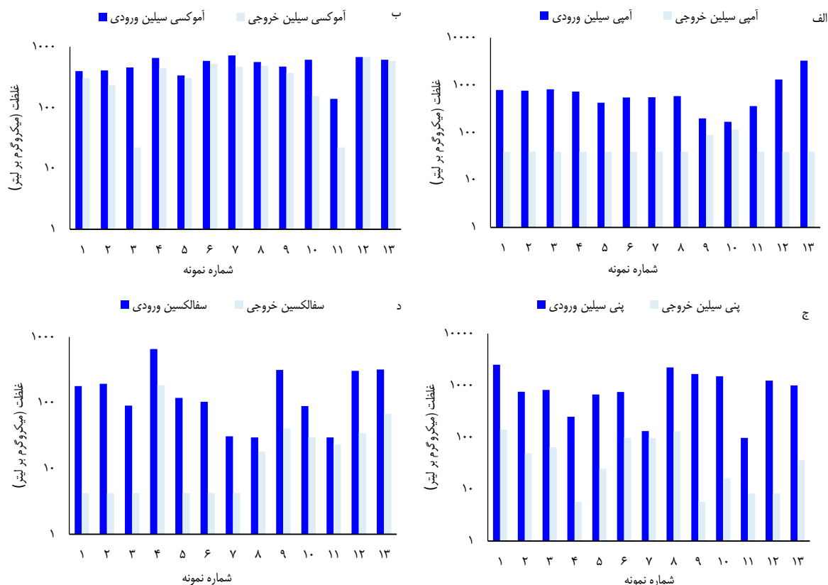
شکل ۳. غلظت آنتی‌بیوتیک در تصفیه‌خانه فاضلاب شرق اصفهان؛ آمپی‌سیلین (الف)، آموکسی‌سیلین (ب)، پنی‌سیلین (ج)، سفالکسین (د)
