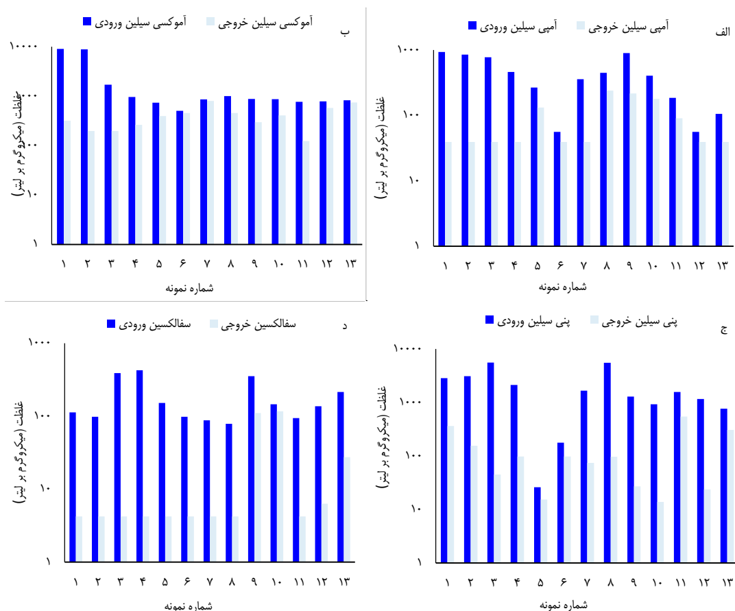
شکل ۴. غلظت آنتی بیوتیک در تصفیه‌خانه فاضلاب جنوب اصفهان: آمپنی سیلین (الف)، آموکسی سیلین (ب)، پنی سیلین (ج)، سفالکسین (د)
