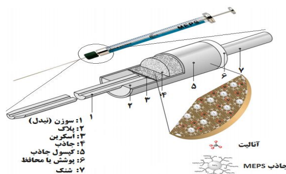
شکل ۱. نمای کلی روش (MEPS) Microextraction by packed sorbent و (MEPS-BIN) MEPS-Barrel Insert and Needle (محفظه بین نیدل و بدنه سرنگ)
