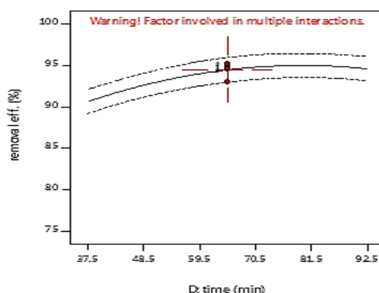
شکل ۹. تأثیر زمان تماس بر راندمان حذف سرب در شرایط نقاط مرکزی سایر متغیرها
