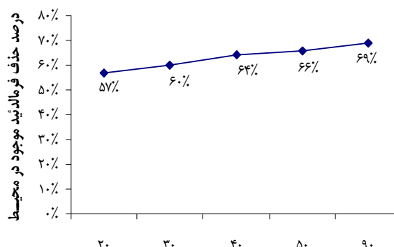
شکل ۲: تغییرات مقدار جذب فرمالدئید در برابر افزایش دمای محیط
