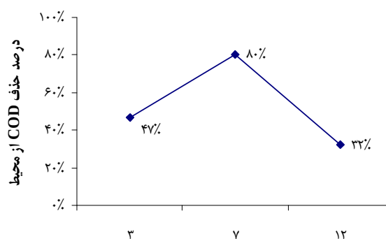
شکل ۳: تغییرات جذب فرمالدئید بر روی موی انسان به واسطه تغییر pH محیط
