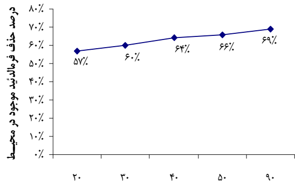
شکل ۲: تغییرات مقدار جذب فرمالدئید در برابر افزایش دمای محیط
