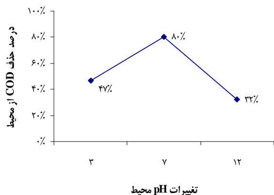
شکل ۳: تغییرات جذب فرمالدئید بر روی موی انسان به واسطه تغییر pH محیط
