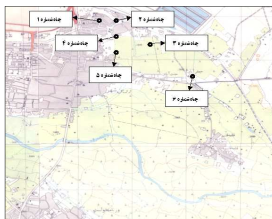
شکل ۱: نقشه محل و موقعیت چاه‌های مورد مطالعه (سجاد زرین شهر)
