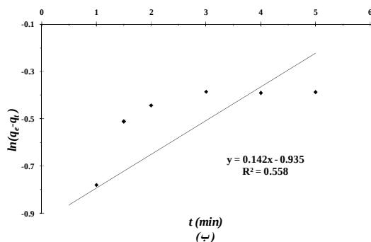
نمودار ۳: سینتیک خطی جذب نیترات با جاذب گرانول هیدروکسید فریک؛ ب) سرعت درجه اول کاذب (لاجرگرن)
