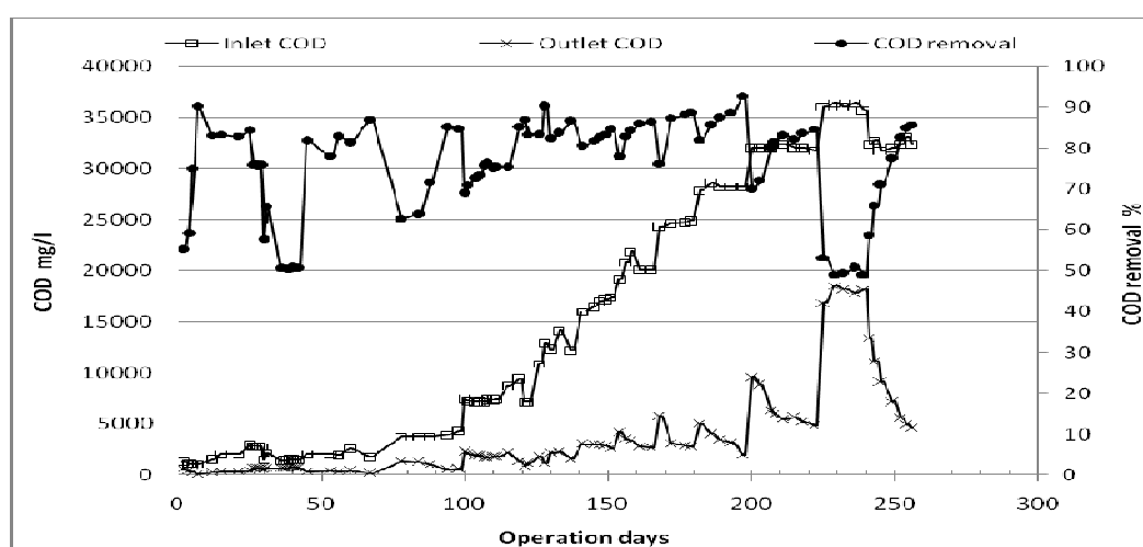
شکل ۳: نمودار بررسی کارایی سیستم در حذف COD
