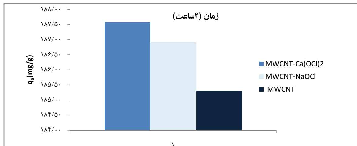
نمودار ۴: ظرفیت جذب بنزن در MWCNT، \text{MWCNT}(\text{Ca}(\text{OCl})_2) و \text{MWCNT}(\text{NaOCl}) با غلظت اولیه ۱۰۰ میلی گرم بر لیتر، غلظت جاذب ۰/۵ گرم بر لیتر و زمان تماس ۲ ساعت MWCNT: Multi walled carbon nano tubes
