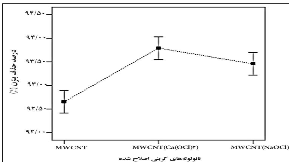
نمودار ۲: درصد حذف بنزن توسط MWCNT، MWCNT(Ca(OCl) 2 ) و MWCNT(NaOCl) با غلظت اولیه ۱۰۰ میلی‌گرم بر لیتر، غلظت جاذب ۰/۵ گرم بر لیتر و زمان تماس ۲ ساعت MWCNT: Multi walled carbon nano tubes
