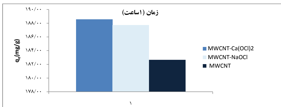
نمودار ۳: ظرفیت جذب بنزن در MWCNT، \text{MWCNT}(\text{Ca}(\text{OCl})_2) و \text{MWCNT}(\text{NaOCl}) با غلظت اولیه ۱۰۰ میلی گرم بر لیتر، غلظت جاذب ۰/۵ گرم بر لیتر و زمان تماس ۱ ساعت MWCNT: Multi walled carbon nano tubes
