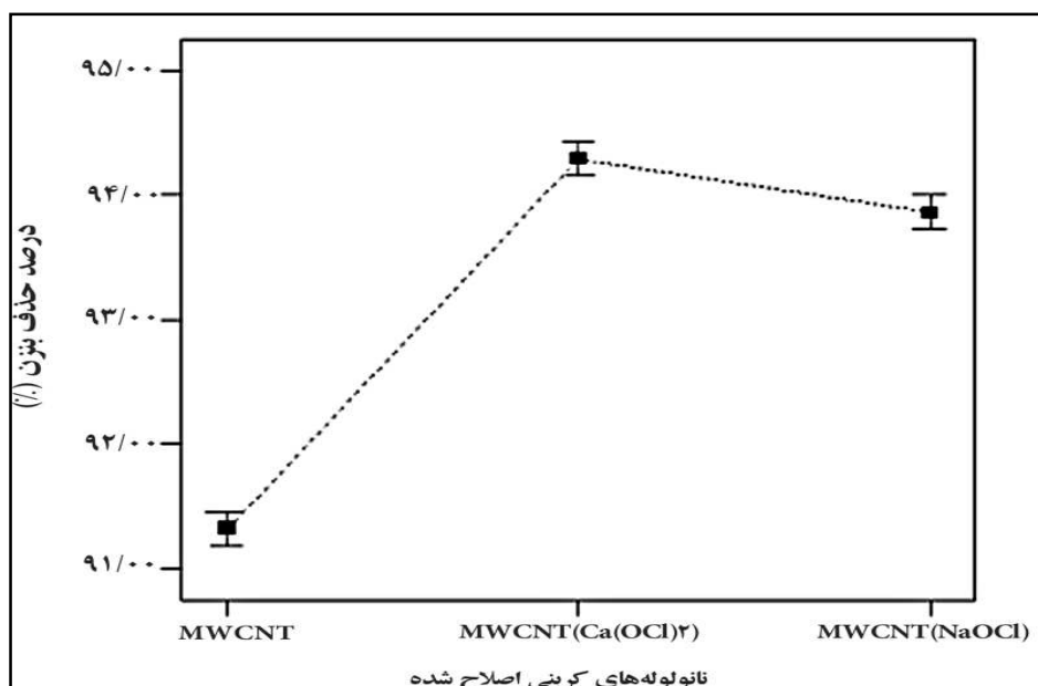
نمودار ۱: درصد حذف بنزن توسط MWCNT، MWCNT(Ca(OCl) 2 ) و MWCNT(NaOCl) با غلظت اولیه ۱۰۰ میلی‌گرم بر لیتر، غلظت جاذب ۰/۵ گرم بر لیتر و زمان تماس ۱ ساعت MWCNT: Multi walled carbon nano tubes
