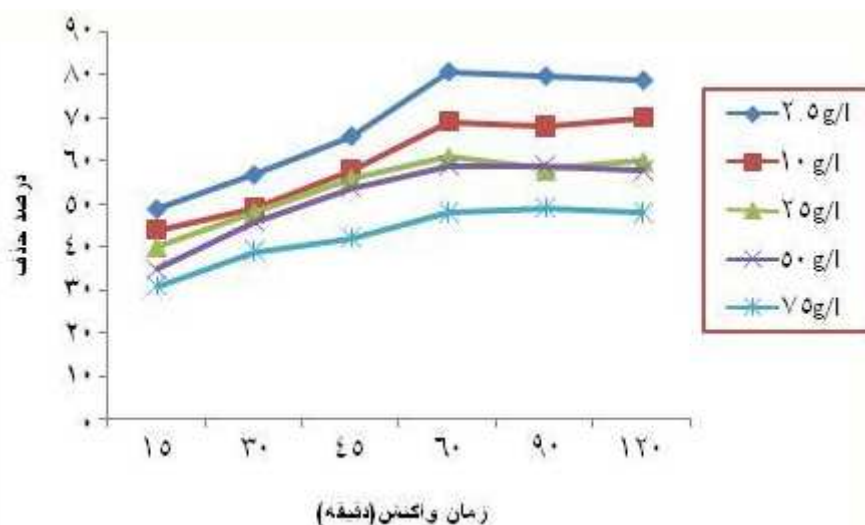
نمودار ۳: تأثیر غلظت اولیه سیانید بر روی میزان حذف سیانید ( \text{pH} = 7 ، مقدار رزین ۳ گرم بر لیتر)
