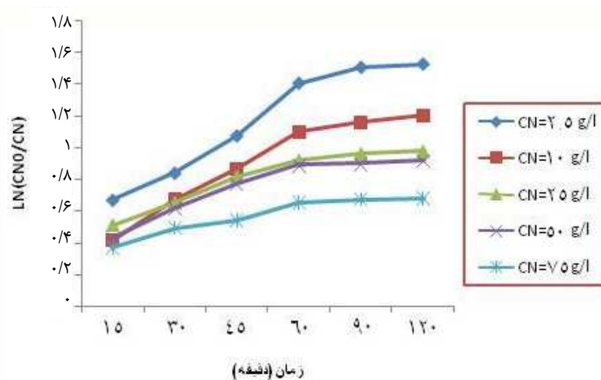
نمودار ۴: نمودار سینتیکی کارایی فرایند حذف سیانید ( pH = 7 ، مقدار رزین ۳ گرم بر لیتر)
