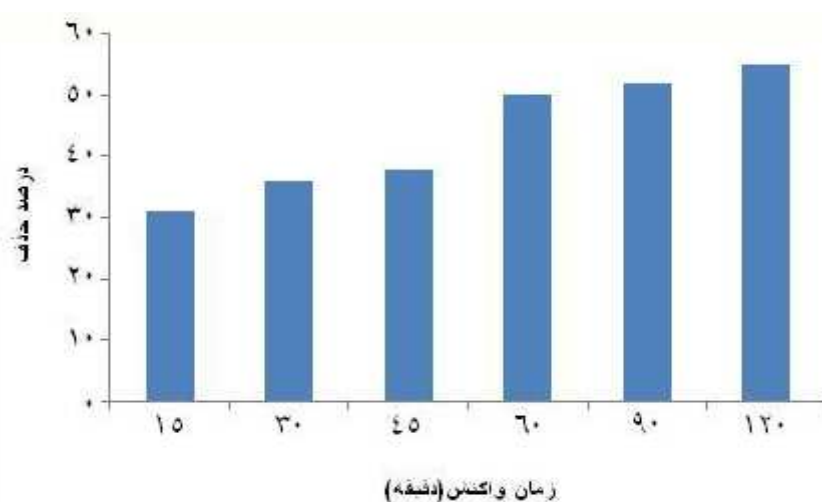
نمودار ۵: تأثیر زمان واکنش بر روی میزان حذف سیانید ( pH = 7 ، مقدار رزین ۳ گرم بر لیتر)
