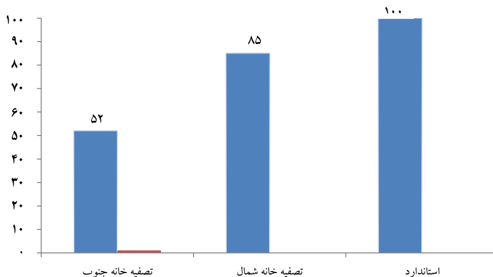
نمودار ۱. مقایسه میانگین مقادیر BOD5 در پساب تصفیه خانه‌های شمال و جنوب اصفهان با استانداردهای محیط زیست ایران
