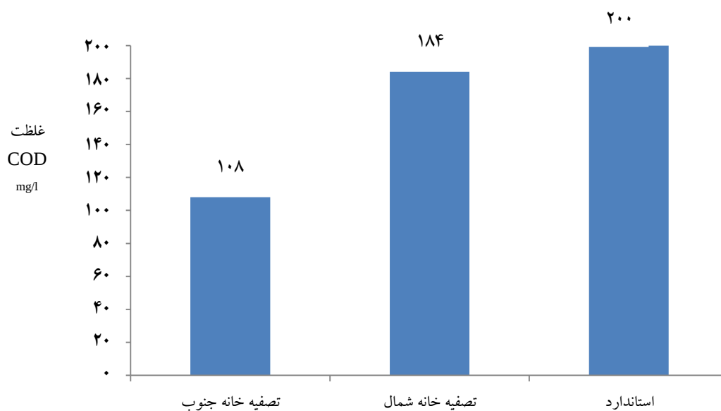
نمودار ۲. مقایسه میانگین مقادیر COD در پساب تصفیه خانه‌های شمال و جنوب اصفهان با استانداردهای محیط زیست ایران
