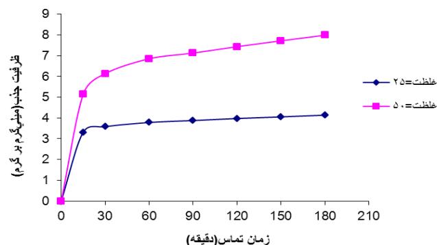
نمودار ۴. ظرفیت جذب رنگ نسبت به زمان با دوز ۰/۶ گرم در لیتر نانولوله کربنی تک جداره (pH=۴) و غلظت های اولیه رنگ ۲۵ و ۵۰ میلی گرم بر لیتر)
