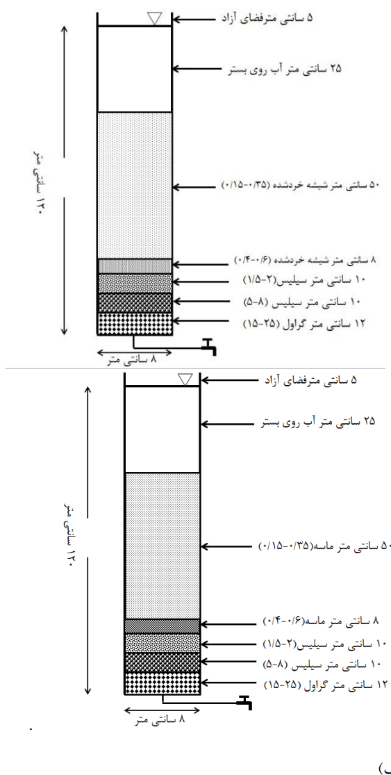
شکل (۱). شماتیک سیستم پایلوت مورد استفاده مطالعه، الف) صافی ماسه‌ای کند متداول (صافی نوع ۱) ب) صافی اصلاح شده با بستر شیشه بازیافتی خرد شده (صافی نوع ۲)
