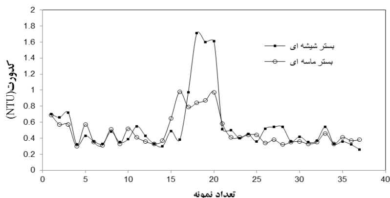
نمودار ۲. نمودار کدورت خروجی از صافی با بستر ماسه‌ای متداول و صافی با بستر شیشه‌ای خردشده بازبافتی در کل دوره نمونه‌برداری
