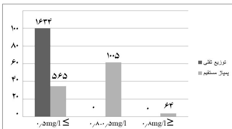
نمودار ۲. میزان کلر باقیمانده در لوله‌ها در دو حالت توزیع ثقیلی و پمپاژ مستقیم
