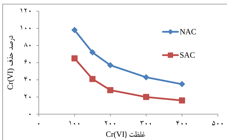
نمودار ۴. راندمان جذب Cr(VI) توسط NAC و SAC در شرایط تعادل (شرایط واکنش: غلظت Cr(VI) ۱۰۰ تا ۴۰۰ میلی‌گرم در لیتر، pH ۲، غلظت جاذب ۱ گرم در لیتر، زمان ۳ ساعت)
