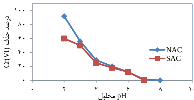
نمودار ۱. اثر pH بر کارایی حذف Cr(VI) (شرایط واکنش: pH ۲ تا ۸، زمان ۳۰ دقیقه، دوز جاذب ۱ گرم در لیتر، غلظت Cr(VI) ۵۰ میلی‌گرم بر لیتر)
