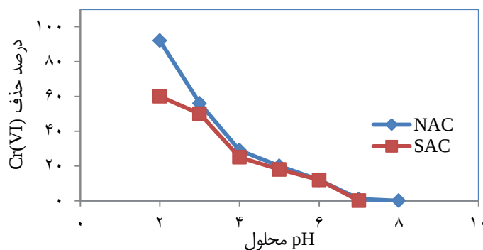
نمودار ۱. اثر pH بر کارآیی حذف Cr(VI) (شرایط واکنش: pH ۲ تا ۸، زمان ۳۰ دقیقه، دوز جاذب ۱ گرم در لیتر، غلظت Cr(VI) ۵۰ میلی‌گرم بر لیتر)
