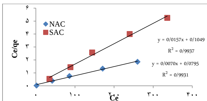
نمودار ۵. ایزوترم جذب لانگمویر نوع ۱ (شرایط واکنش: غلظت Cr(VI) ۱۰۰ تا ۴۰۰ میلی گرم در لیتر، pH ۲، دوز جاذب ۱ گرم در لیتر، زمان ۱۸۰ دقیقه)
