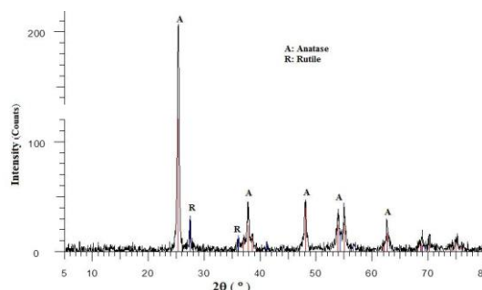
شکل ۲. الگوی XRD نانوذرات \text{TiO}_2
