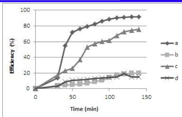
شکل ۵. راندمان حذف فتوکاتالیستی با غلظت 10 \text{ mg/L} (a) \text{TiO}_2/\text{Zeolite} با شدت تابش 3/9 \text{ w/m}^2 (b) \text{TiO}_2 با شدت تابش 3/9 \text{ w/m}^2 ؛ (c) \text{TiO}_2/\text{Zeolite} با شدت تابش 2/4 \text{ w/m}^2 (d) \text{TiO}_2 با شدت تابش 2/4 \text{ w/m}^2
