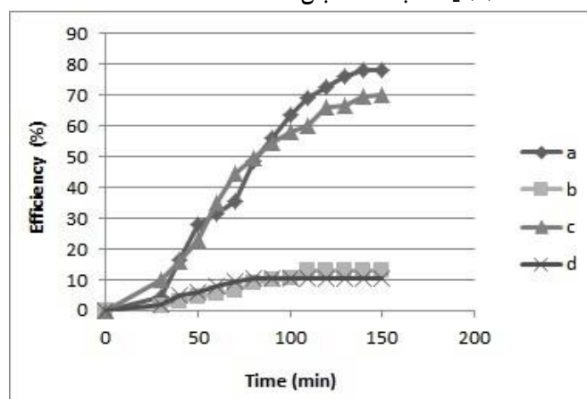
شکل ۶. راندمان حذف فتوکاتالیستی با غلظت 50 \text{ mg/L} (a) \text{TiO}_2/\text{Zeolite} با شدت تابش 3/9 \text{ w/m}^2 (b) \text{TiO}_2 با شدت تابش 3/9 \text{ w/m}^2 ؛ (c) \text{TiO}_2/\text{Zeolite} با شدت تابش 2/4 \text{ w/m}^2 (d) \text{TiO}_2 با شدت تابش 2/4 \text{ w/m}^2
