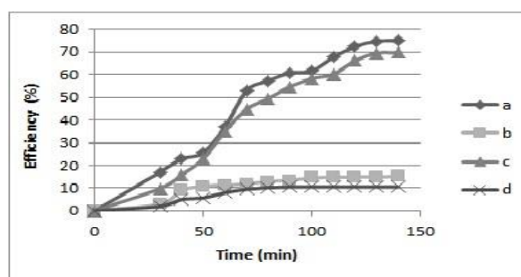
شکل ۴. راندمان حذف فتوکاتالیستی (a) \text{TiO}_2/\text{Zeolite} با غلظت ۱۰ mg/L؛ (b) \text{TiO}_2 با غلظت ۱۰ mg/L؛ (c) \text{TiO}_2/\text{Zeolite} با غلظت ۵۰ mg/L؛ (d) \text{TiO}_2 با غلظت ۵۰ mg/L
