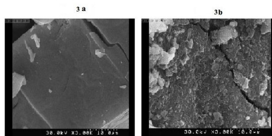
شکل ۳. (a) الگوی SEM نانوذرات \text{TiO}_2 - شکل (b) الگوی SEM \text{TiO}_2/\text{Zeolite}
