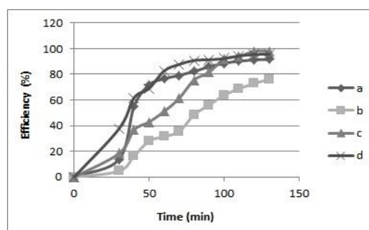
شکل ۸. راندمان حذف کاتالیستی با 3/9 \text{ w/m}^2 شدت تابش فرابنفش (a) بستر ثابت \text{TiO}_2/\text{Zeolite} با غلظت ۱۰ \text{mg/L} ؛ (b) بستر ثابت \text{TiO}_2/\text{Zeolite} با غلظت ۵۰ \text{mg/L} ؛ (c) بستر متحرک \text{TiO}_2/\text{Zeolite} با غلظت ۱۰ \text{mg/L} ؛ (d) بستر متحرک \text{TiO}_2/\text{Zeolite} با غلظت ۵۰ \text{mg/L}
