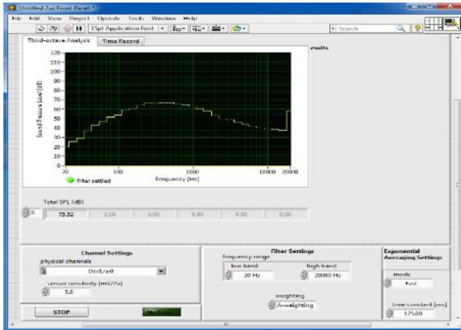
شکل ۶. اندازه‌گیری تراز فشار صوت در یک سوم اکتاواند
