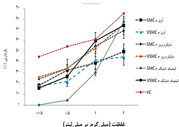
شکل ۳. مقایسه میانگین اثر بستر کشت و روش خشک کردن بر اثر بازداری در غلظت های مختلف عصاره SMC: کمپوست برگشتی قارچ VSMC: ورمی کمپوست
