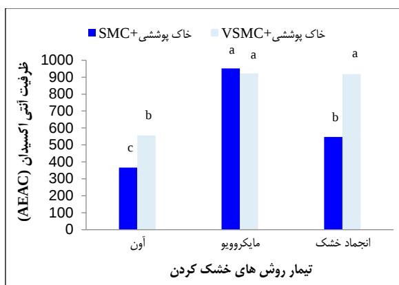
شکل ۲. مقایسه میانگین اثر ترکیبی بستر کشت × روش خشک کردن بر ظرفیت آنتی اکسیدان (AEAC) میانگین هایی که حداقل یک حرف مشترک دارد، اختلاف معنی داری در سطح ۵ درصد آزمون Duncan ندارد. SMC: کمپوست برگشتی قارچ، VSMC: ورمی کمپوست
