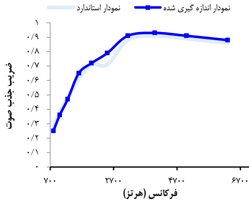
شکل ۱. مقایسه ضرایب جذب استاندارد با مقادیر اندازه‌گیری شده فوم استاندارد با ضخامت ۲۵ میلی‌متر
