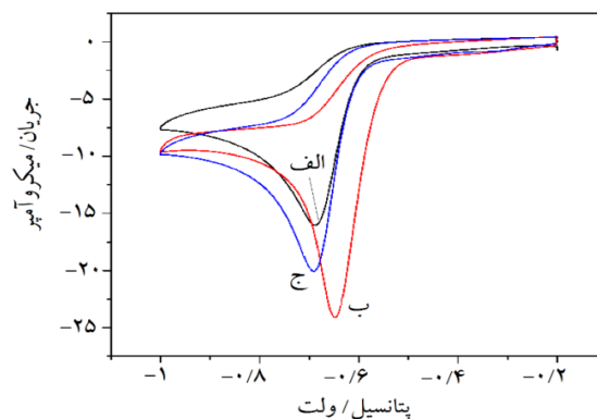
شکل ۶. ولتاموگرام‌های چرخه‌ای الکتروکود اصلاح شده با نانوذرات نیکل اکسید جریان ۵۰ میلی‌آمپر (الف)، ۱۰۰ میلی‌آمپر (ب) و ۵۰۰ میلی‌آمپر (ج) در زمان ۳۰ ثانیه با وجود ۱۰۰ میکرومولار پارانیتروفنل در محلول بافر فسفات و pH = ۷ و سرعت روبش ۲۰ میلی‌ولت بر ثانیه
