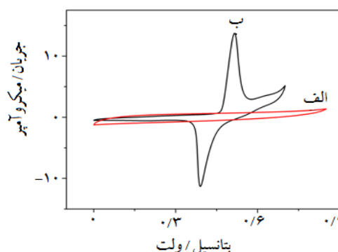
شکل ۴. ولتاموگرام‌های چرخه‌ای الکتروکربن شیشه‌ای (الف) و الکتروکربن شیشه‌ای اصلاح شده با نانوذرات نیکل اکسید (ب) در محلول ۰/۱ مولار سدیم هیدروکسید در سرعت روبش ۵۰ میلی ولت بر ثانیه
