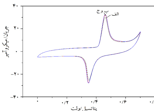
شکل ۵. ولتاموگرام‌های چرخه‌ای الکتروکربن شیشه‌ای اصلاح شده با فیلم نانوساختار نیکل اکسید در دومین (الف)، صد و پنجاهمین (ب) و صد و پنجاهمین (ج) چرخه پتانسیل اعمالی به الکتروکربن (محلول ۰/۱ مولار هیدروکسید سدیم و سرعت روبش ۱۰۰ میلی ولت بر ثانیه)
