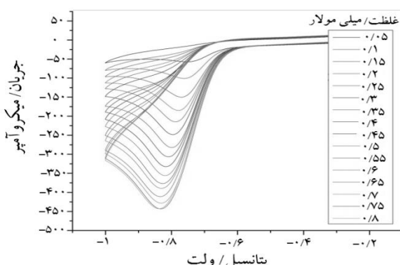
شکل ۵. ولتاموگرام‌های چرخه‌ای الکتروکود اصلاح شده با فیلم نانوساختار نیکل اکسید در غلظت‌های متفاوت ۵۰، ۱۰۰ و... تا ۸۰۰ میکرومولار از پارانیتروفنل در محلول بافر فسفات با pH = ۷ و سرعت روبش ۲۰ میلی‌ولت بر ثانیه
