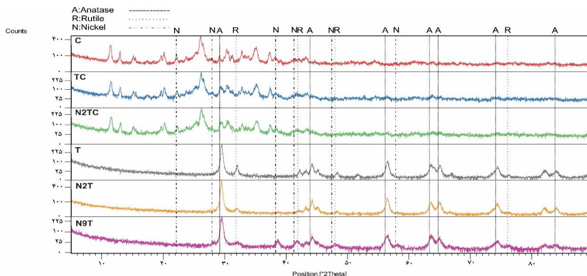
شکل ۱. مقایسه زئولیت کلینوپتیلولیت خالص (C) (قرمز)، TC (آبی)، N_7TC (سبز)، TiO_2 خالص (T) (خاکستری)، T_1N (نارنجی) و N_1T (بنفش)
