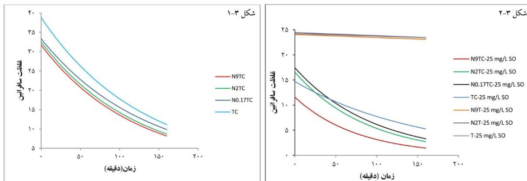
شکل ۳. تغییرات غلظت ۵۰ و ۲۵ میلی گرم بر لیتر سافرانین نسبت به زمان زمان صفر: ثابت شدن غلظت سافرانین بر اثر جذب سطحی و روشن شدن لامپ UV
