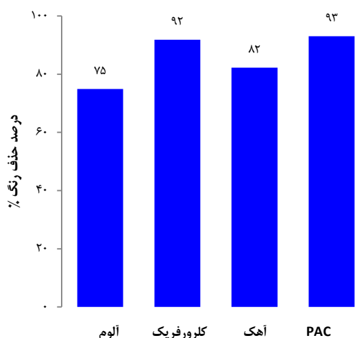
شکل ۱. مقایسه‌ای راندمان‌های حذف رنگ و COD برای منعقد
