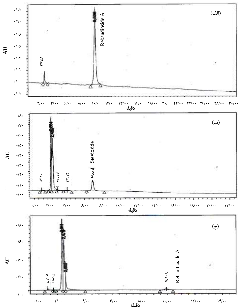
شکل ۱. کروماتوگرام high performance liquid chromatography (HPLC) مربوط به (الف) محلول استاندارد ۱۰۰ \mu\text{g/ml} ربودیوزید A، (ب) محلول استاندارد ۱۰۰ \mu\text{g/ml} استویوزید (ج) نمونه منتخب استویا (شرایط دستگاهی: ستون C_{18} ، درجه حرارت ۴۰ درجه سلسیوس، فاز متحرک آب- استونیتریل (۸۰:۲۰)، سرعت جریان ۱ میلی‌لیتر/دقیقه و طول موج ۲۱۰ نانومتر)
