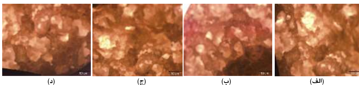
شکل ۲. تصاویر میکروسکوپ نوری فوم‌های نانوکامپوزیت پلی استایرن/ خاک رس. (الف) فوم پلیمر استایرن، (ب) فوم پلی استایرن/ خاک رس ۰/۵ درصد، (ج) فوم پلی استایرن/ خاک رس ۳ درصد، (د) فوم پلی استایرن/ خاک رس ۷ درصد
