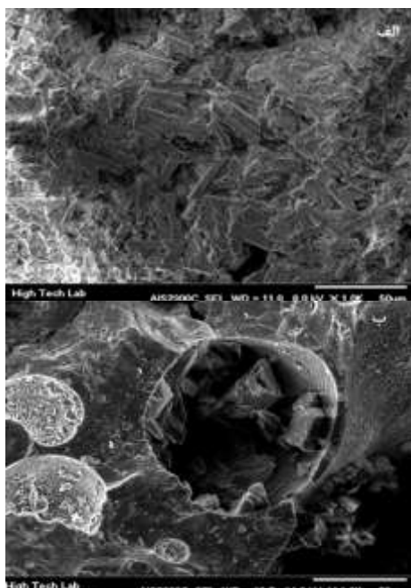
شکل ۳. نمای SEM (Scanning electron microscope) پامیس طبیعی (الف) و اصلاح شده (ب) بعد از جذب آلایند
