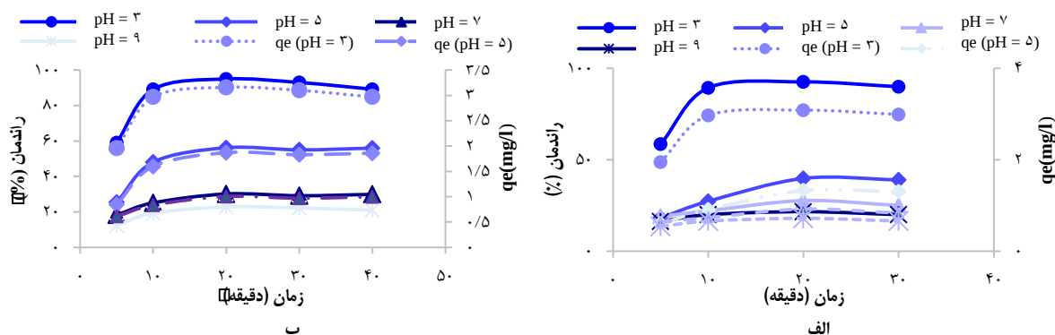
شکل ۴. تأثیر pH و زمان تماس بر راندمان و ظرفیت جذب با استفاده از پامیس طبیعی (الف) و پامیس اصلاح شده (ب) (دوز جذب ۳۰ گرم در لیتر و غلظت ۱۰ میلی گرم بر لیتر)
