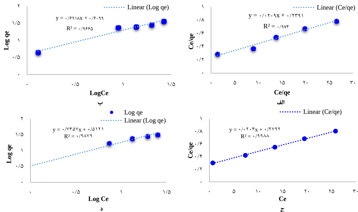
شکل ۷. ایزوترم Langmuir و Freundlich برای پامیس طبیعی (الف، ب) و ایزوترم Langmuir و Freundlich برای پامیس اصلاح شده (ج، د)
