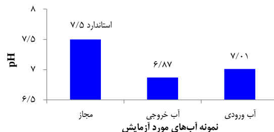
شکل ۲. مقایسه مقدار pH ورودی و خروجی با مقدار مجاز آب آشامیدنی
