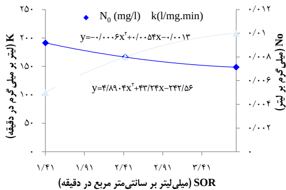
شکل ۲. ضریب سرعت و ظرفیت جذب کروم شش ظرفیتی با استفاده از ستون‌های جاذب (Granular activated carbon) GAC بر حسب بار سطحی
