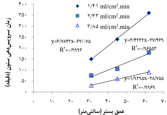
شکل ۱. زمان کارکرد ستون‌های جاذب (Granular activated carbon) بر حسب تغییرات عمق ستون
