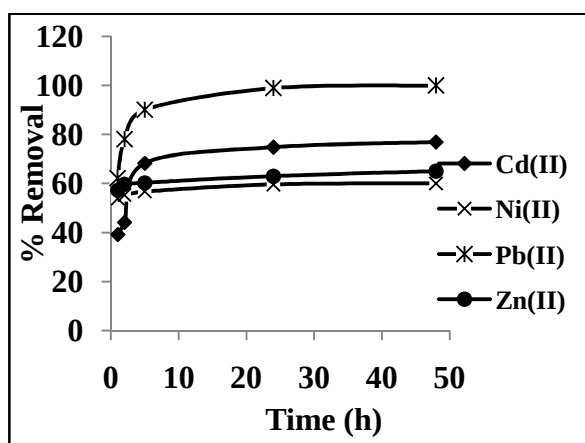
نمودار ۲: اثر زمان تماس بر درصد جذب کاتیون فلزات سنگین توسط سیلیکا آئروژل اصلاح شده بهینه برای هر pH، ۴۰۰ mg/L، غلظت = ۵۰ mL (حجم = ۰/۵ g کاتیون، جذب)
